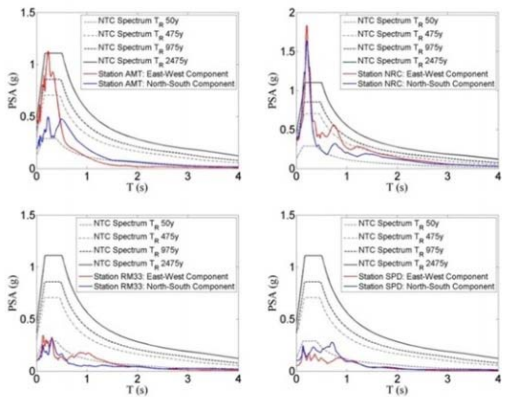
Figura 6: Spettri di risposta orizzontali osservati e spettri di norma per quattro periodi di ritorno per le quattro stazioni più vicine all'epicentro. Da sopra, in senso antiorario: AMT (distanza 8,9 km), NRC (distanza 13,7 km), RM33 (distanza 22,3 km), SPD (distanza 23,7 km)
